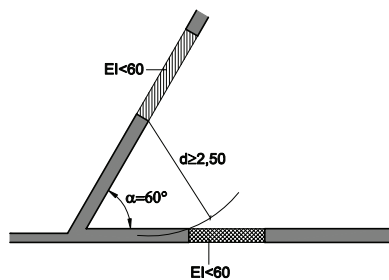
Figura 1.3. Fachadas a 60°
