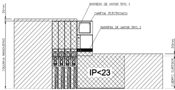
ALZADO
