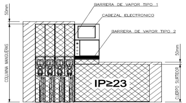
ALZADO
